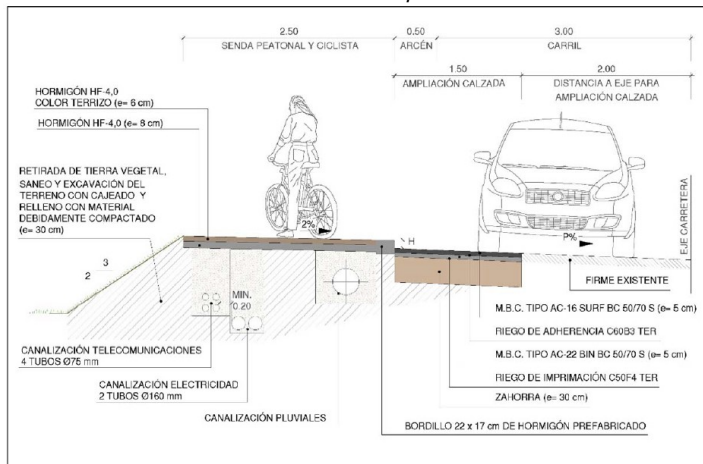
Sección transversal da senda
